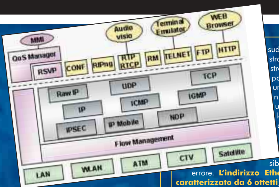
Lo stack di Internet.
