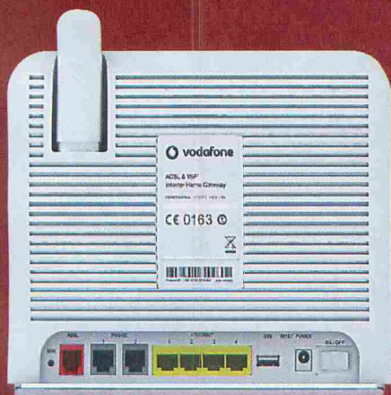
▲ Figura 1: la VS oltre ad avere molte porte monta un processore dual-core MIPS da 300MHz, 64Mb di RAM e 16Mb flash.
